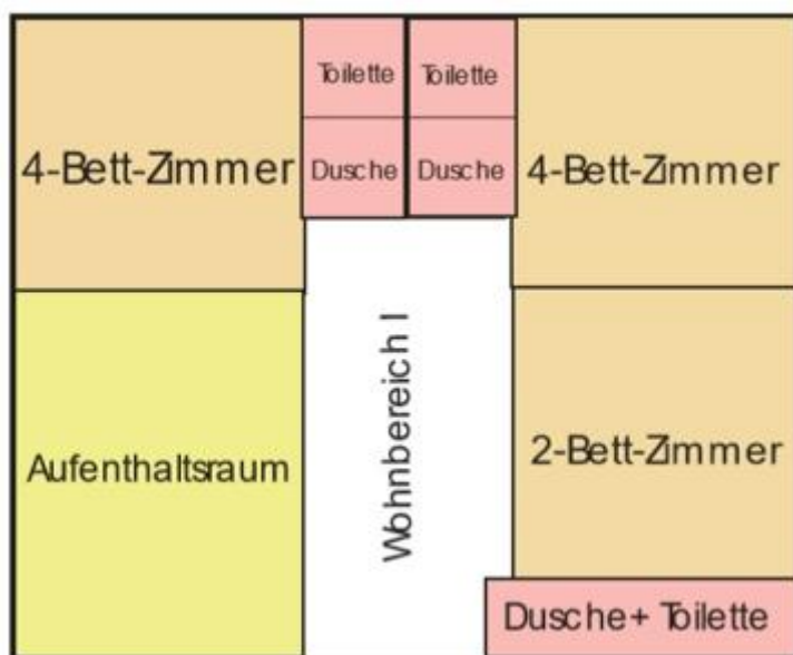
Grundriss der Ferienhäuser
